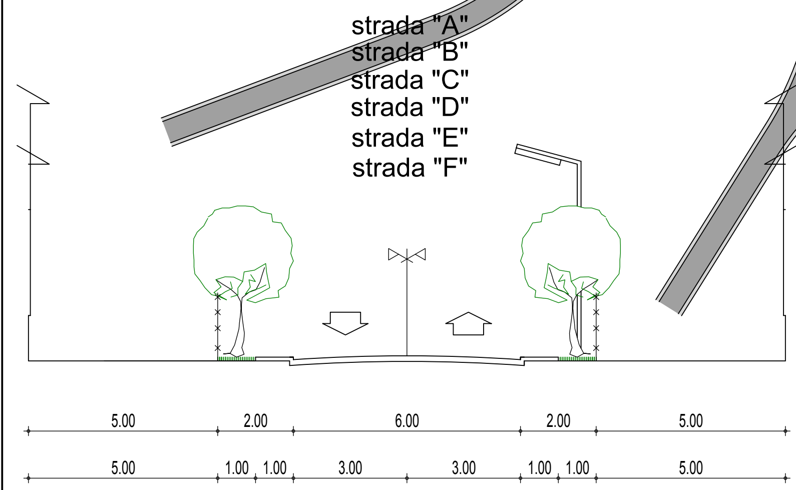
profil "A-A"
