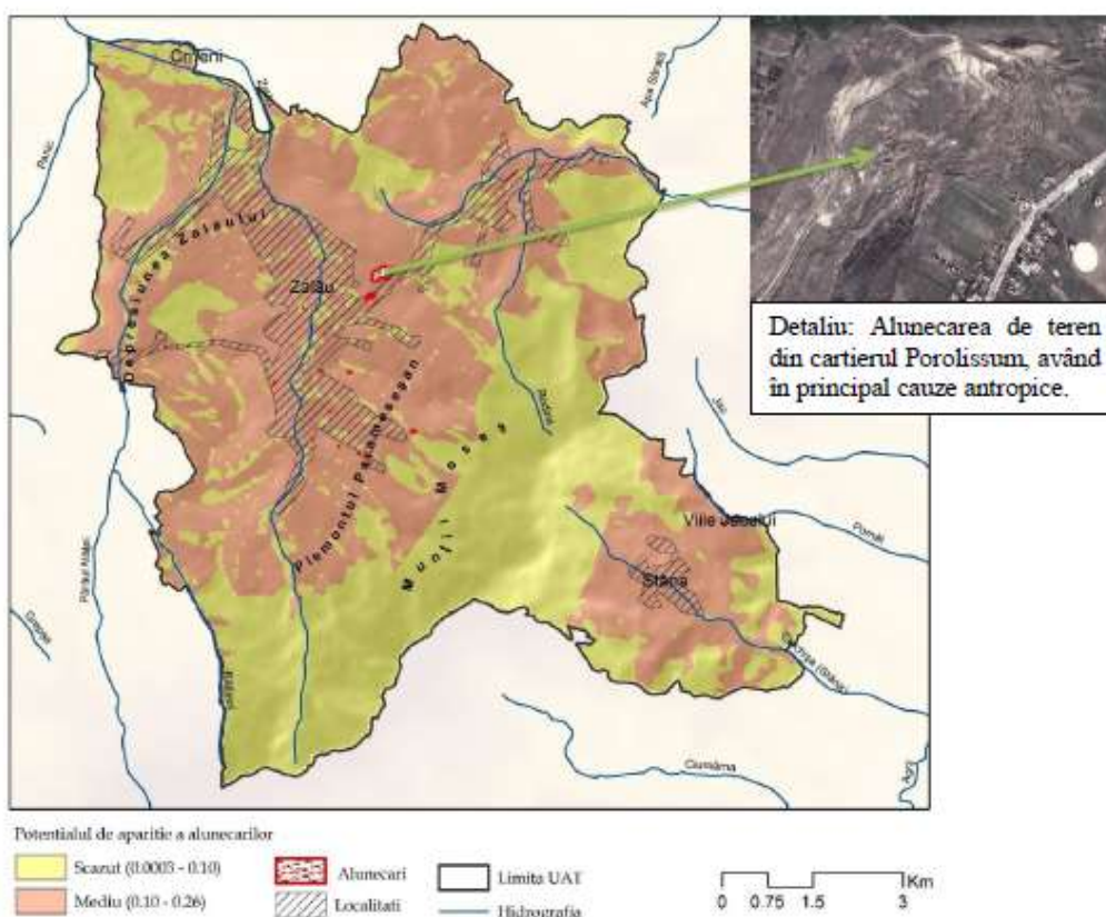
Harta 2: Alunecări de teren active pe clase de probabilitate
